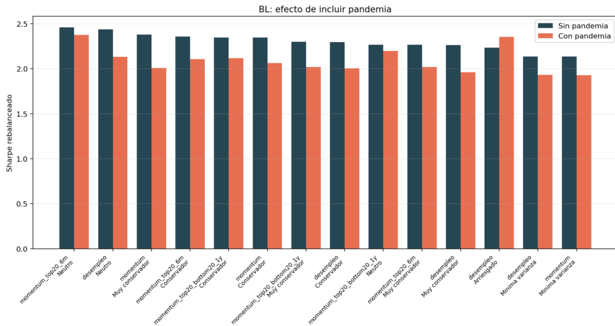
Figura 9. Efecto de pandemia en views Black-Litterman.
