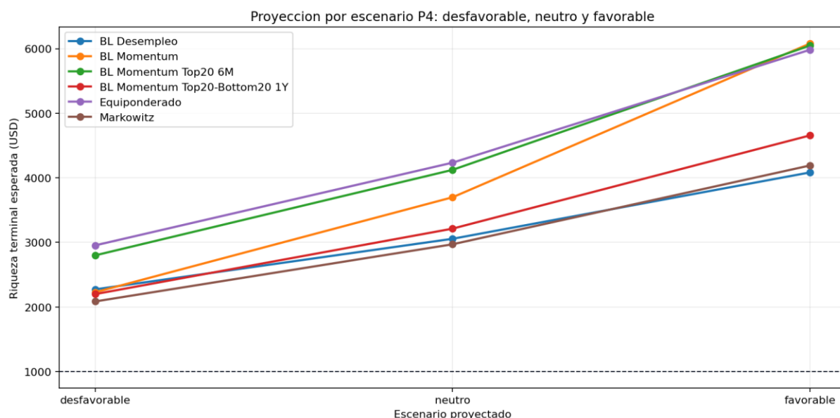
Figura 16. Sensibilidad por escenario proyectado.
