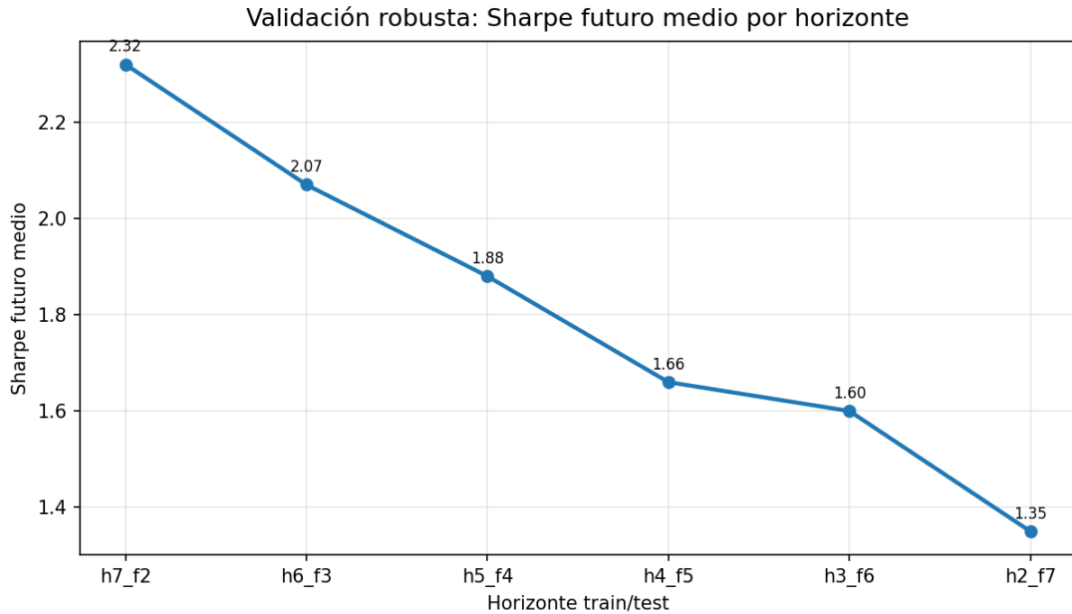
Figura 7. Validacion robusta de Sharpe por horizonte.
